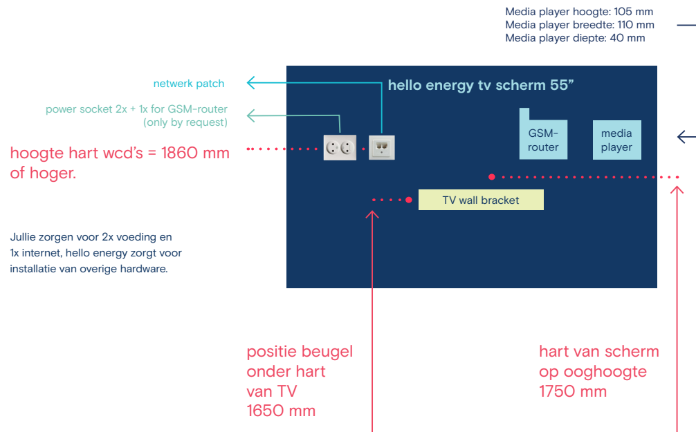
Schets van de achterzijde van een 55" horizontaal scherm na de installatie.
